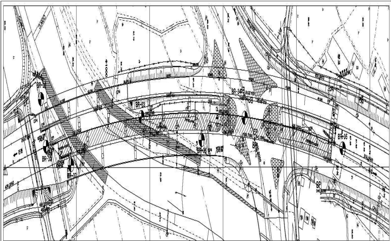
【그림 1.1.1】 죽산1교(상행_용인방향) 평면도
