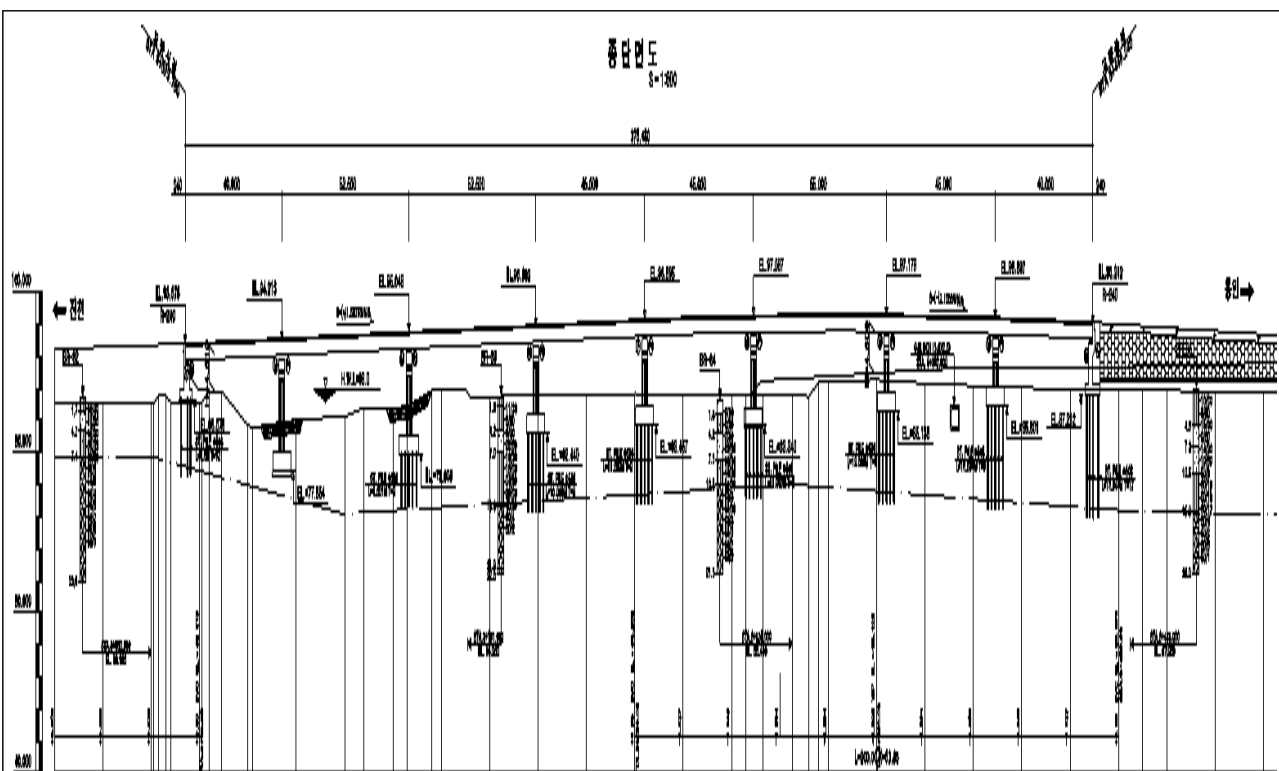
【그림 1.1.2】 죽산1교(상행_용인방향) 종단면도
