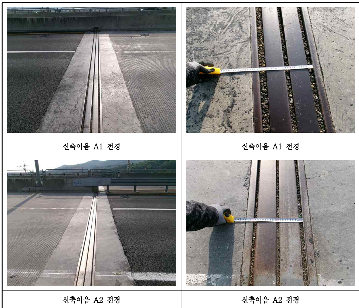
【사진 1.2.3】 신축이음장치 현황
