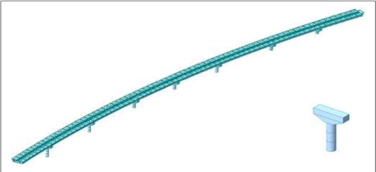
【그림 1.4.1】 축산1교(상행_용인방향) 교량 구조해석 모델링
